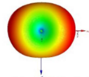
Curved Dipole 1.3 dBi (+z)
