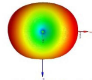
Curved Dipole 1.3 dBi (+z)
